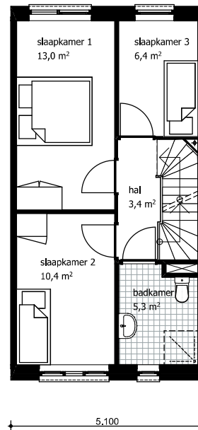
GO 1e verdieping 43,7 m 2
