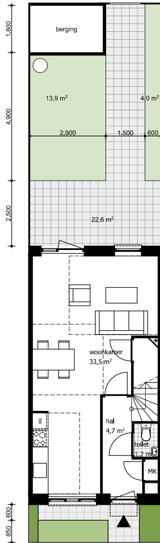
GO begane grond 43,7 m 2
