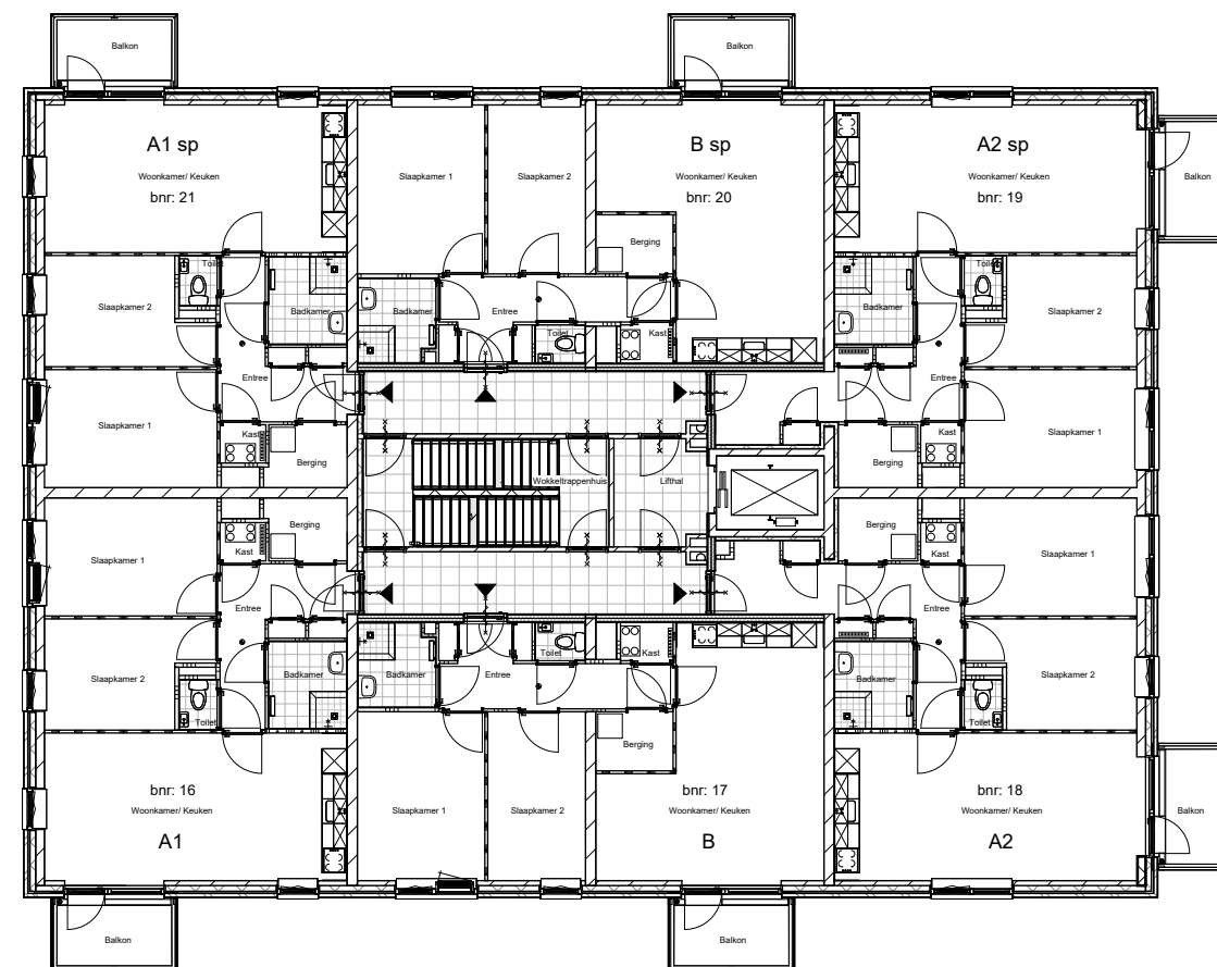
3e verdieping
