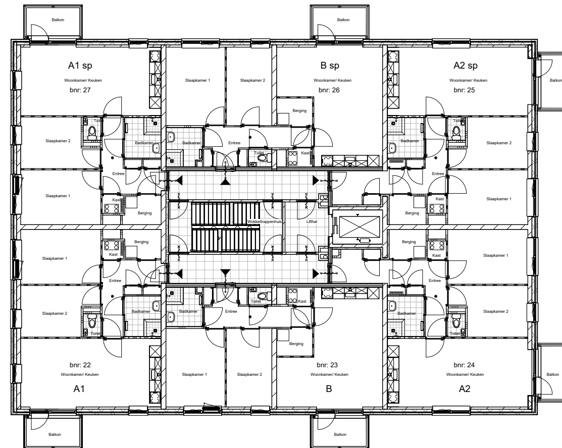
4e verdieping
