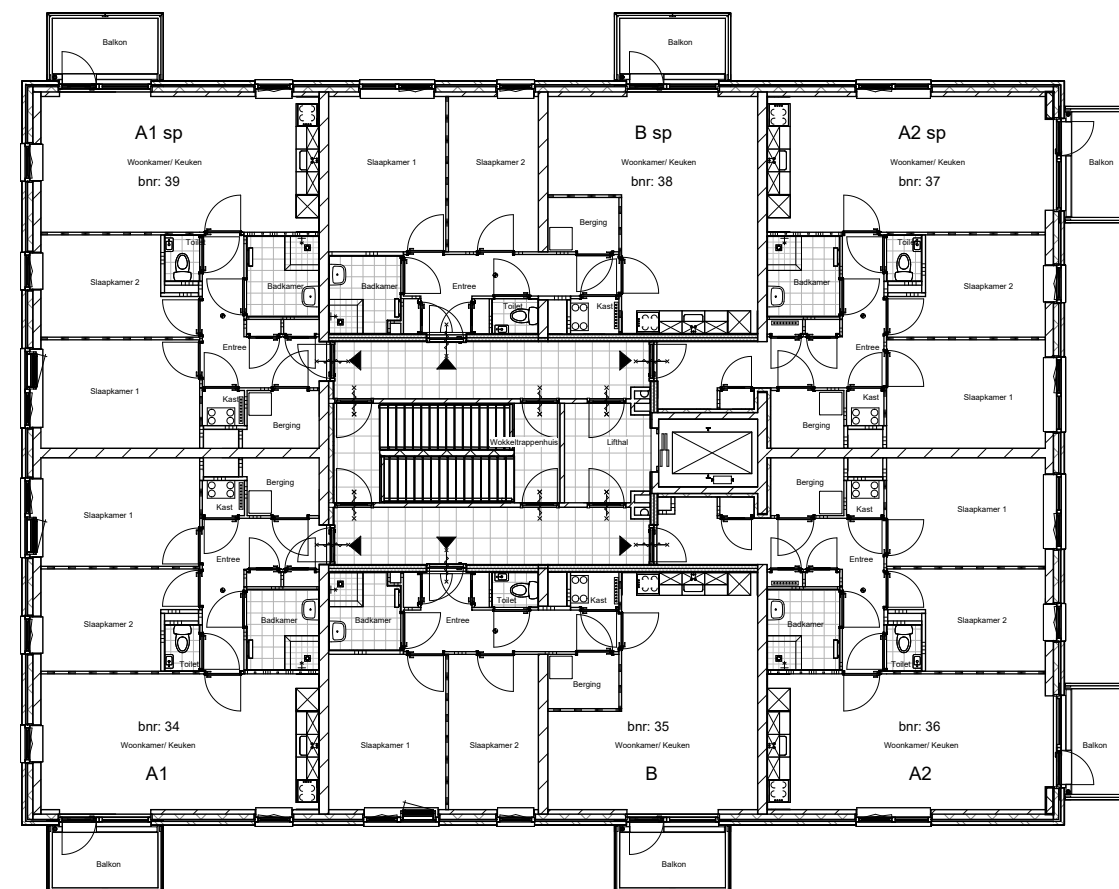
6e verdieping
