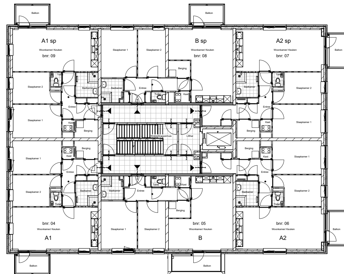
1e verdieping
