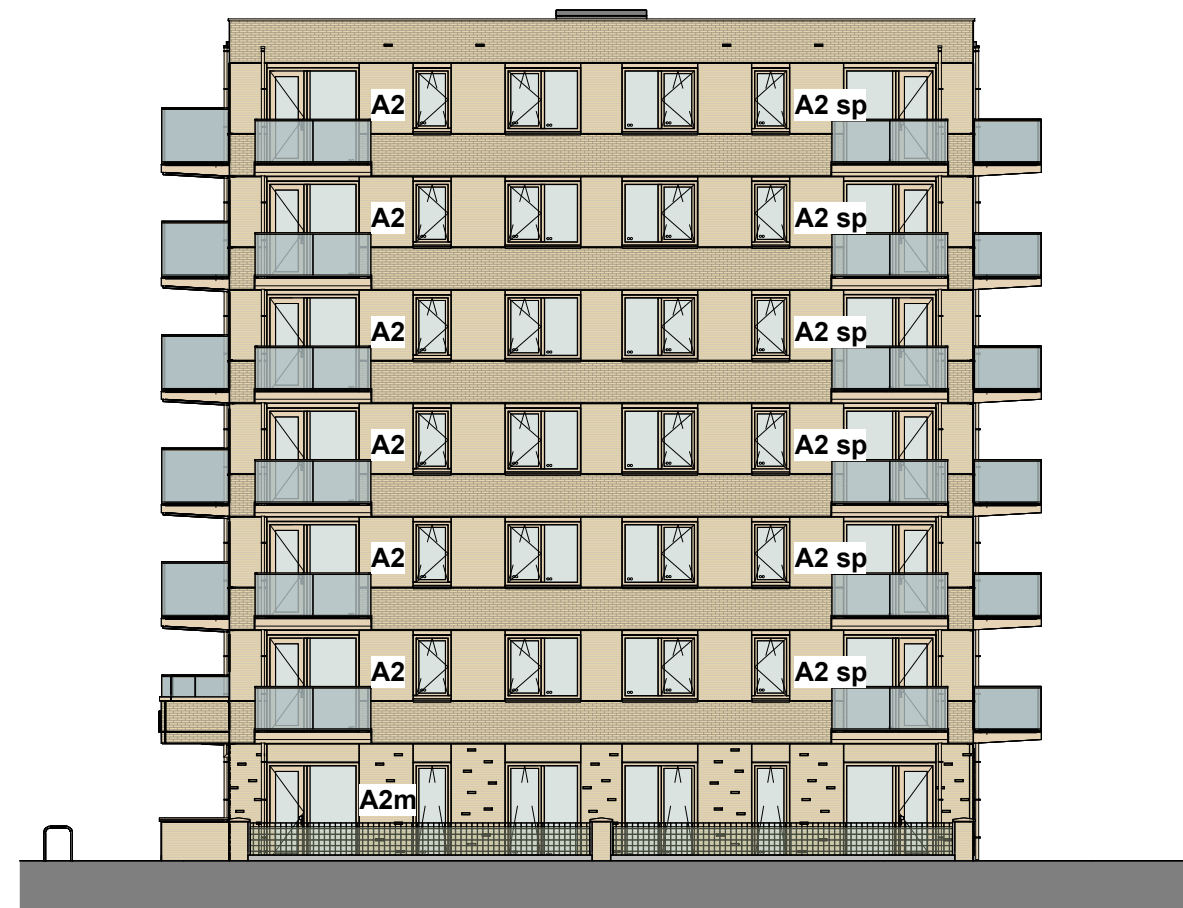
Rechter zijgevel
