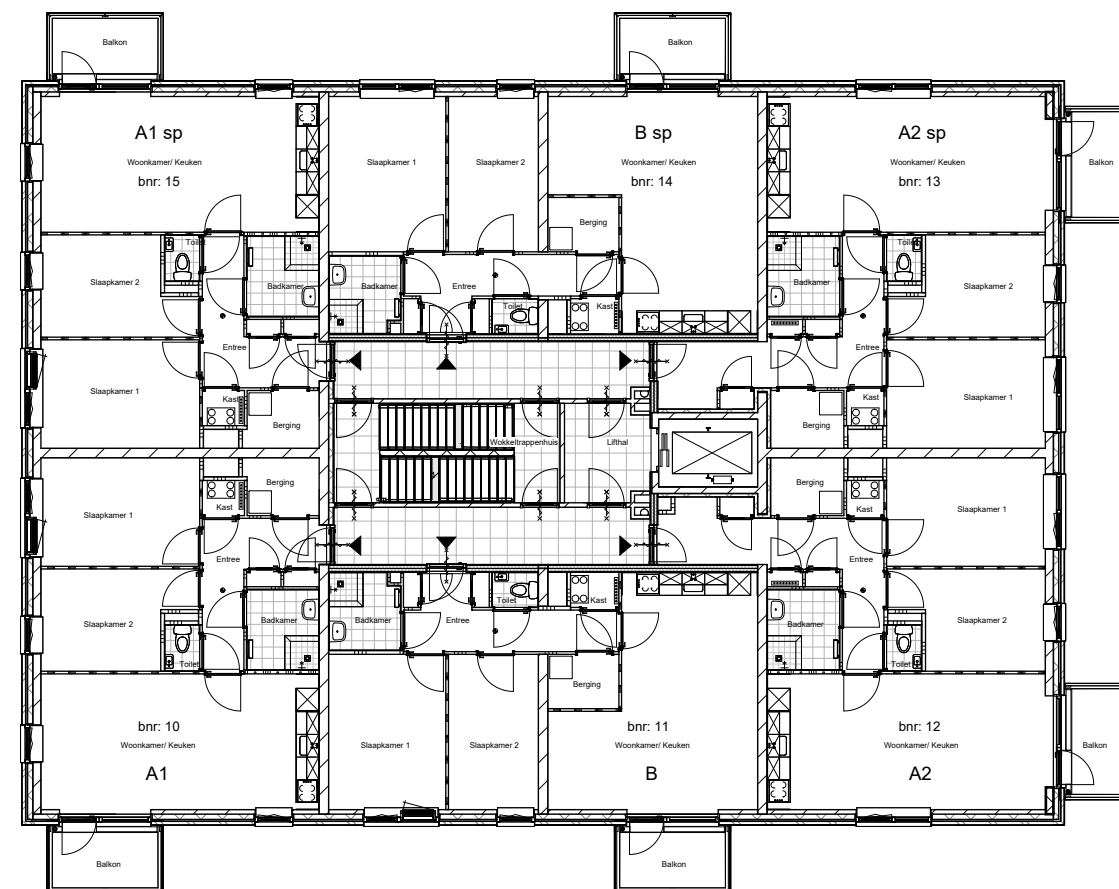
2e verdieping
