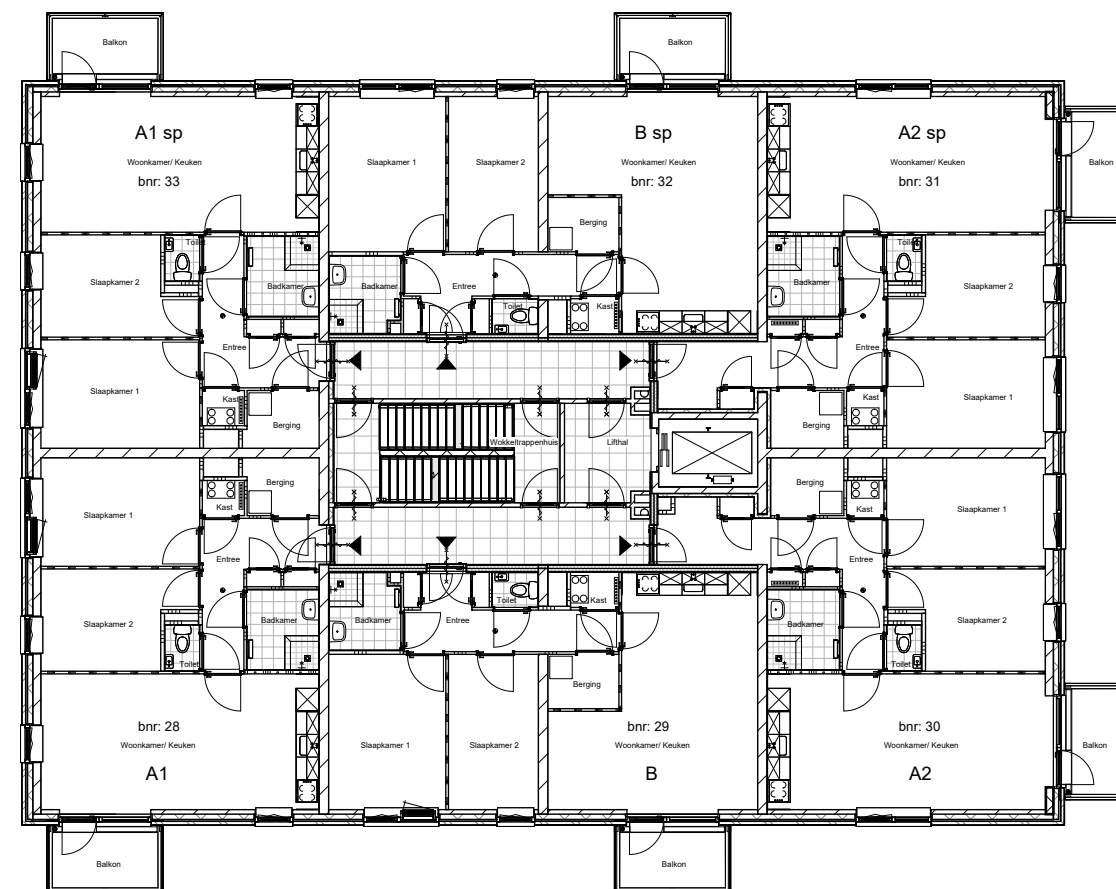
5e verdieping
